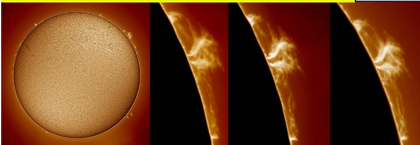
Aspecte de la cromosfera el 15 de gener de 2011, on la major part de manifestacions actives tenen lloc a l'hemisferi nord. Cal destacar una protuberància pel NO, de la qual podem observar en detall a les tres imatges de la dreta i la seua evolució en poc menys d'una hora a les 11:30. Imatges de José Muñoz Reales des de Barcelona amb Lumenera.
