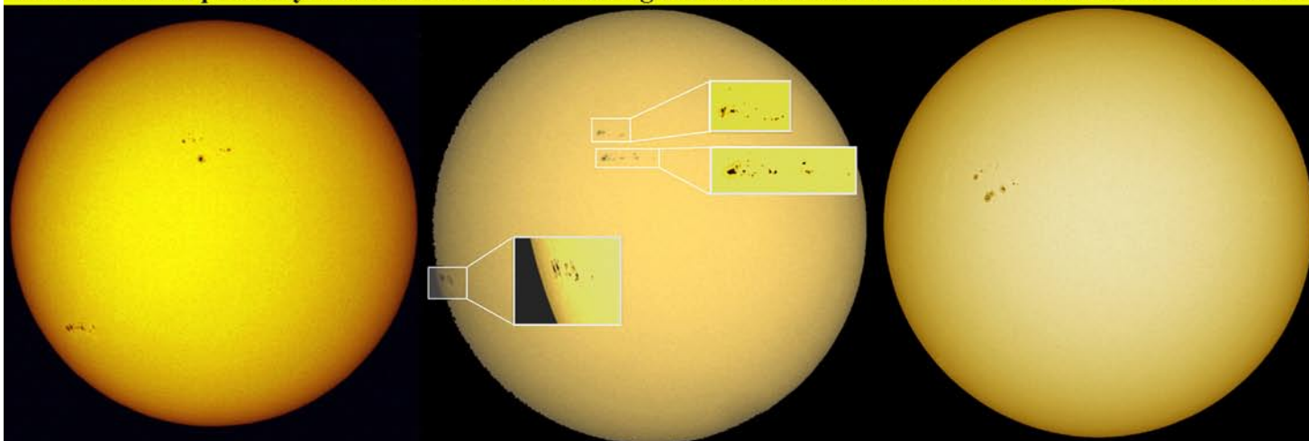
La fotosfera ha pres gran protagonisme pel que fa a la cromosfera, destacant nombrosos grups durant els dies 8 i 23 de febrer, assolint-se valors del número de Wolf força elevats front al llarg mínim d'aquests anys arrere. Les imatges són dels dies 18, 19 i 20, fetes per Joan M. Bullon, Fabio Mariuza i Javier Temprano respectivament.
