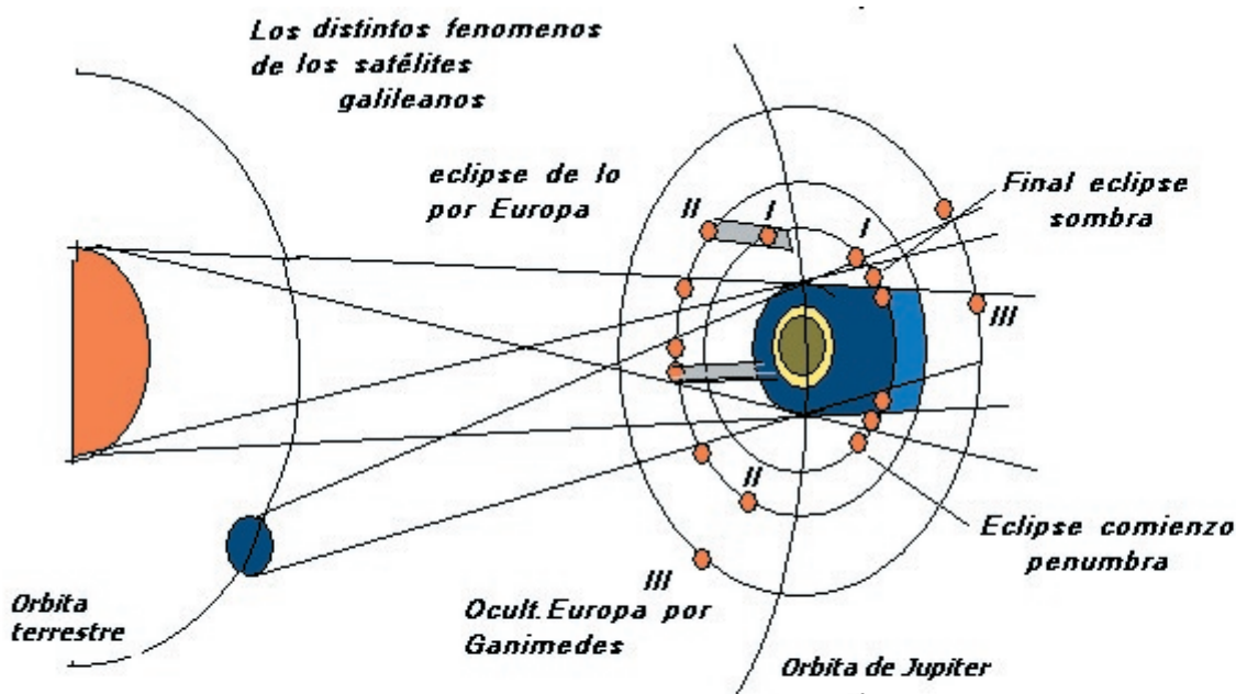
Esquema de los fenómenos clásicos y mutuos de los satélites de
