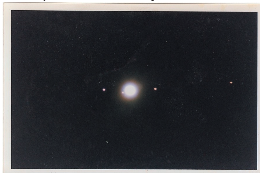
Los "galileanos" orbitando a Júpiter
